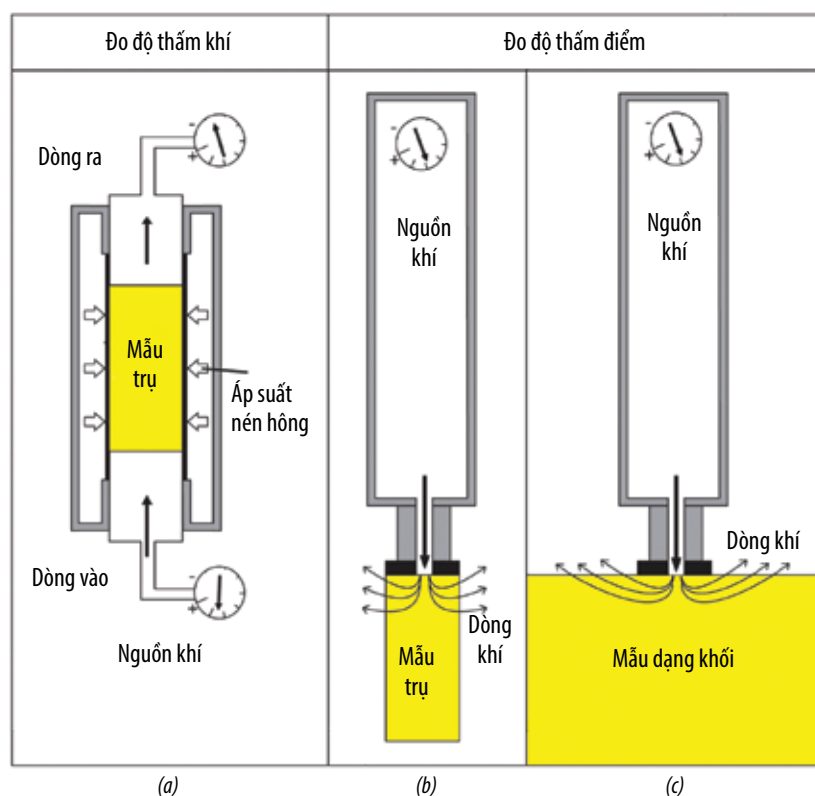
Hình 1. Mô hình dòng chảy qua mẫu khí đo độ thấm khí (a) và khí đo độ thấm điểm (b, c) [2].
