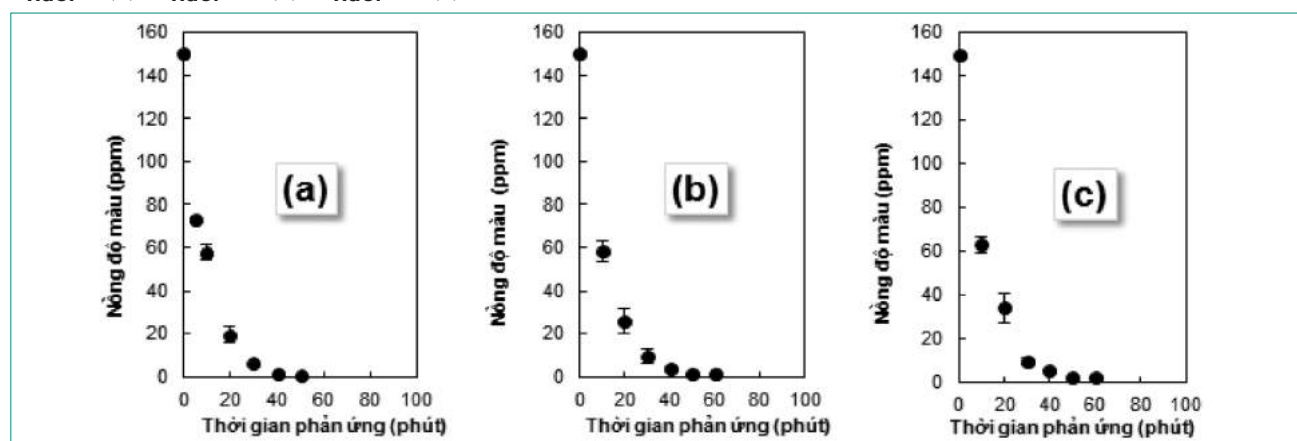
Hình 5. Ảnh hưởng của nồng độ NaCl trong dung dịch xử lý đối với hiệu quả xử lý màu nước thải bằng ozone bột mịn tại: m_{NaCl}=0 (a), m_{NaCl}=1\% (b), m_{NaCl}=3\% (c)
