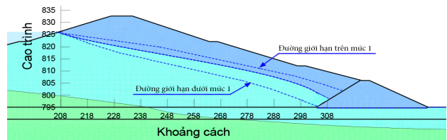
Hình 4. Kết quả xác định các đường bão hòa giới hạn của mức 1 ứng với MNDBT
