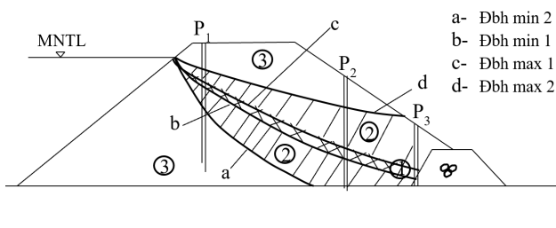
Hình 1. Các mức giới hạn của đường bảo hòa ứng với một mực nước thượng lưu.
