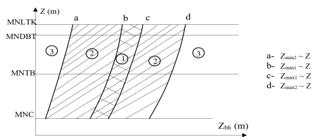
Hình 2. Biểu diễn các đường giới hạn của đường bảo hòa trong thân đập đất (tại 1 điểm)
